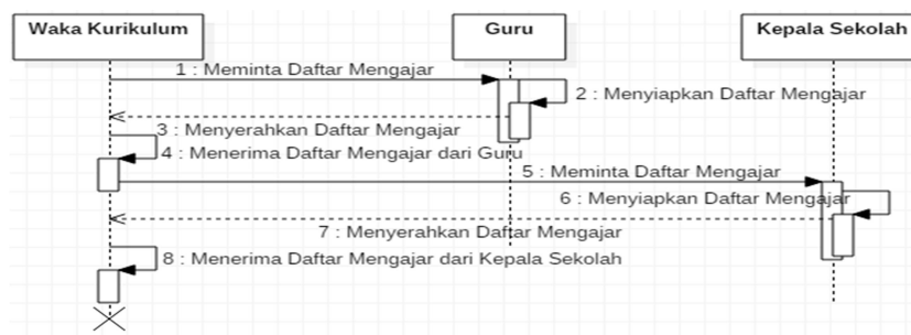
Gambar 3. Diagram Sekuensial Pengumpulan Data Sistem yang Diusulan
