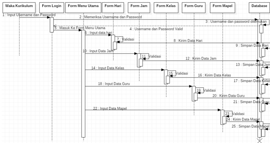
Gambar 4. Diagram Sekuensial Input Data Sistem yang Diusulan
