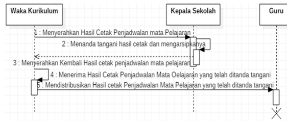
Gambar 6. Diagram Sekuensial Pembuatan Laporan Sistem yang Diusulan
