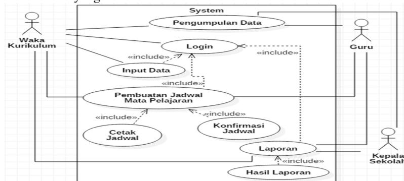
Gambar 1. Diagram Use Case Sistem yang Diusulkan
