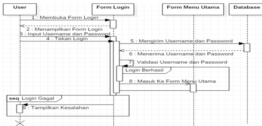
Gambar 2. Diagram Sekuensial Login Sistem yang Diusulan
