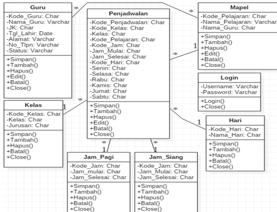
Gambar 7. Diagram Kelas
